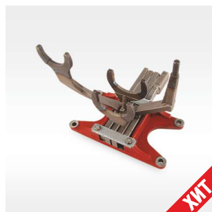
КОРПУС ВИЛОК КОРОБКИ ПЕРЕДАЧ
